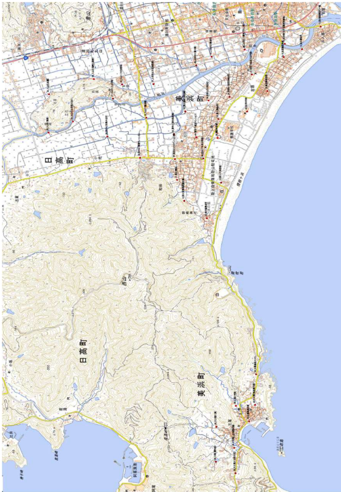
IV-5 同報系無線システム配置図
